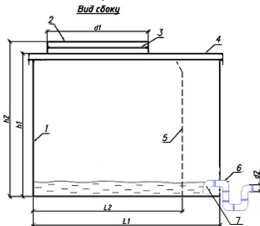
Рисунок 1 - Схема пескоуловителя
